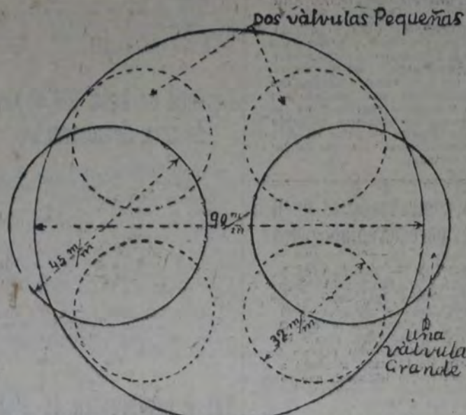
Diagrama comparativo del espacio ocupado por válvulas grandes y pequeñas montadas sobre las culatas del cilindro
